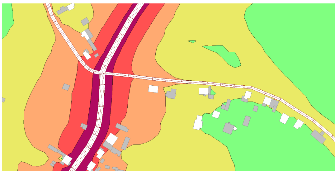
♦ Rysunek 36: Przykładowy zasięg stref hałasu drogowego [widok z oprogramowania CADNA]
