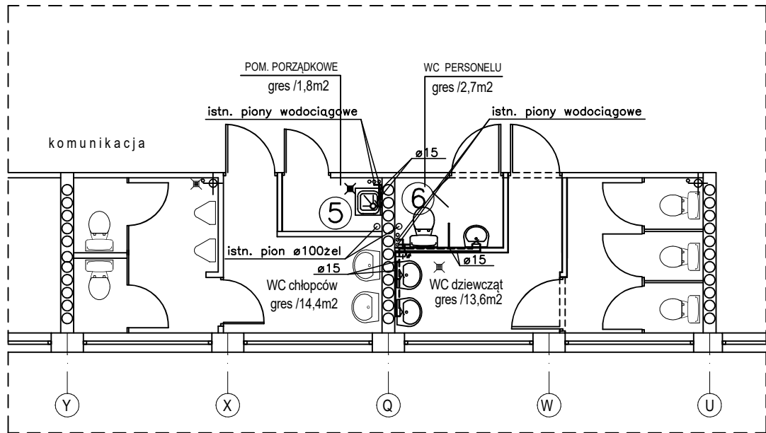
WĘZŁY HIGIENICZNO SANITARNE SEGMENT "C" - Ip i IIp
